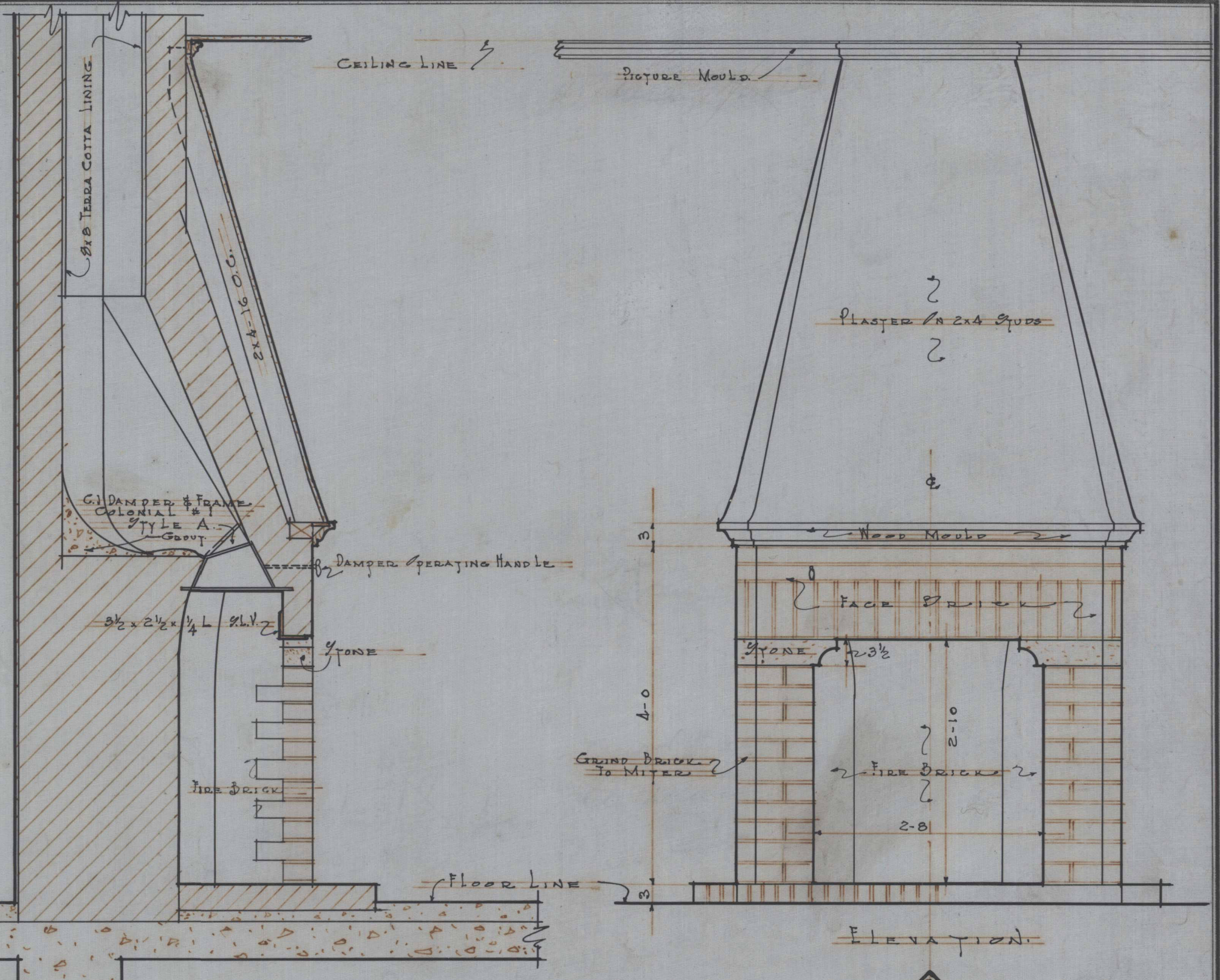
SECTION A-C
